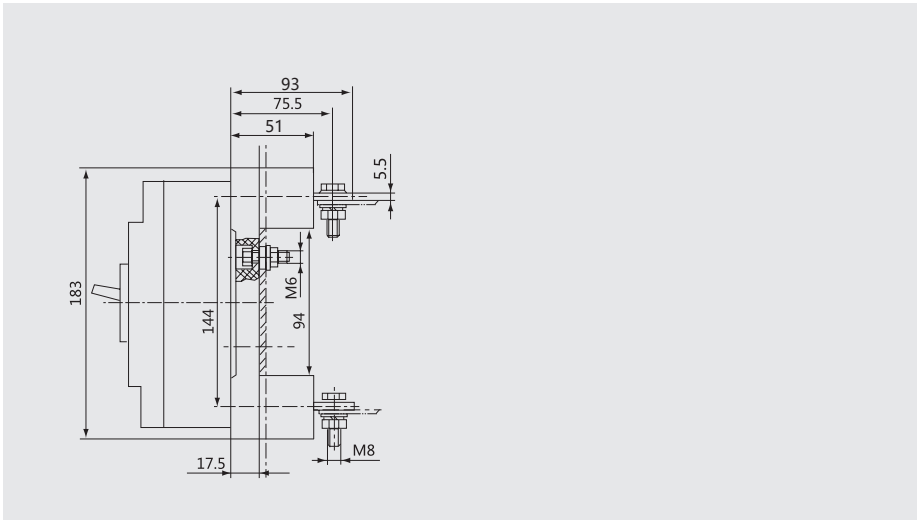
Z2H：插入式板后接线（二极、三极）（X-X、Y-Y为断路器中心）
