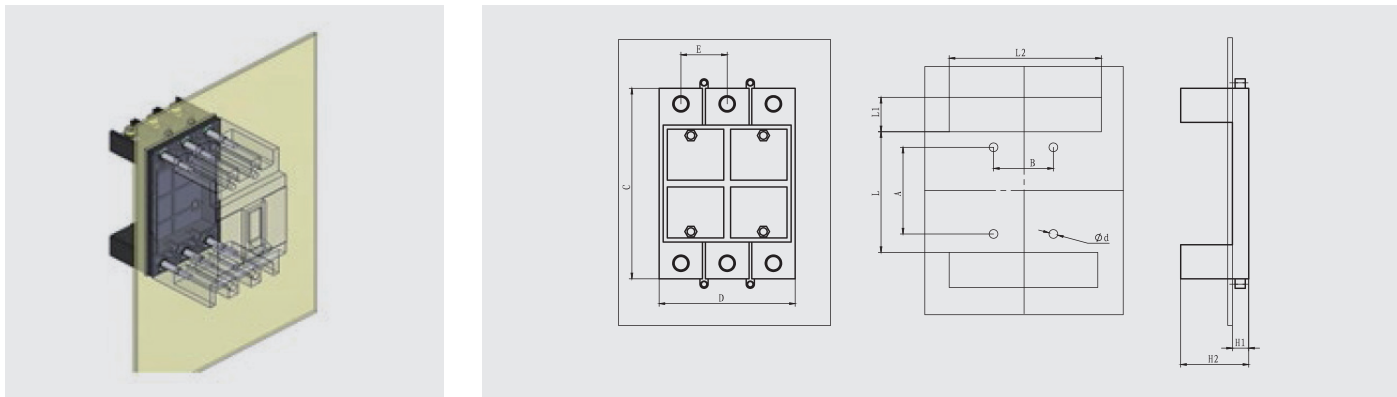
安装示意图：
