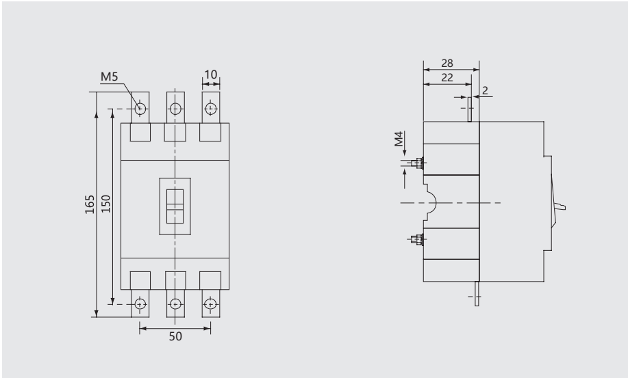
Z2Q：插入式板前接线（二极、三极）（X-X、Y-Y为断路器中心）
