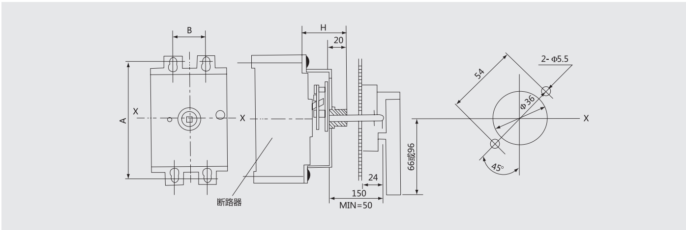
CS1-F型手柄安装开孔示意图
