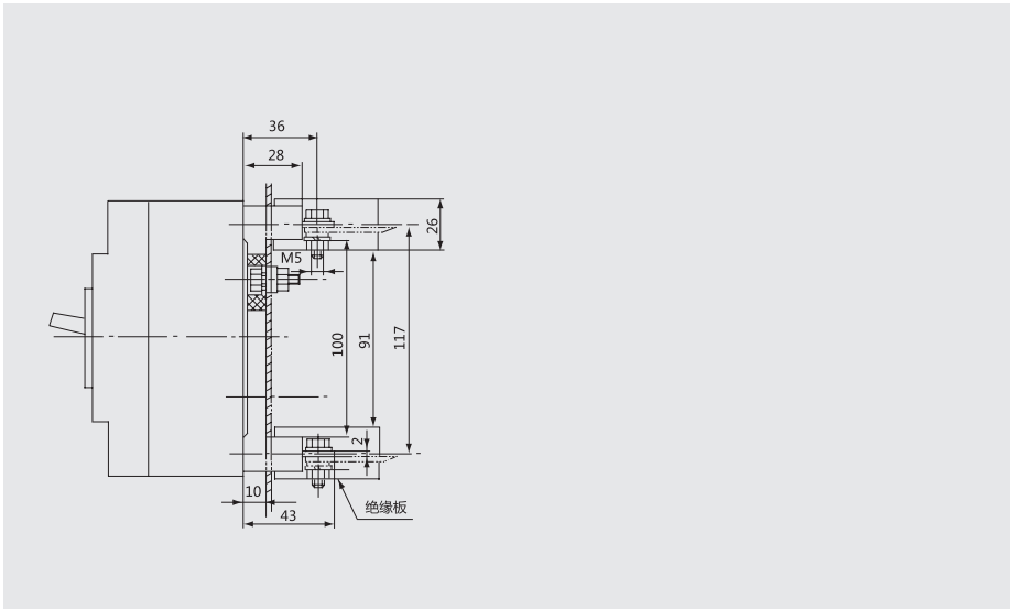
Z2H：插入式板后接线（二极、三极）（X-X、Y-Y 为三极断路器中心）
