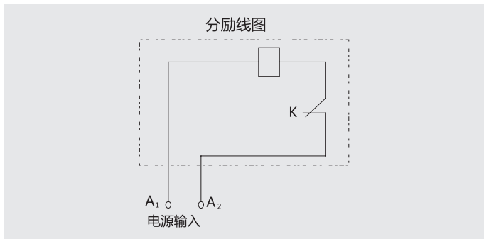
分励脱扣器接线图
