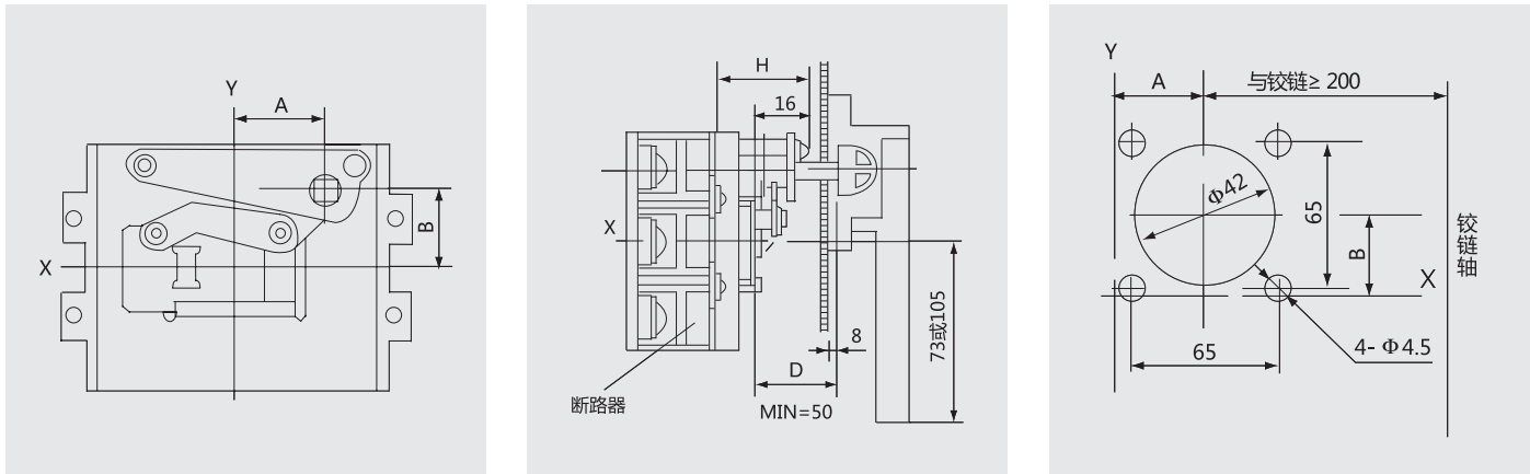
手动操作机构的安装方法及其外形尺寸
