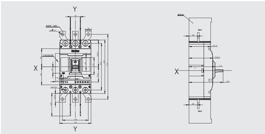
板前接线（X-X、Y-Y为三极断路器中心）
