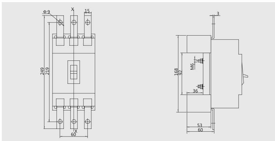
Z2Q: 插入式板前接线 (二极、三极) (X-X、Y-Y为断路器中心)
