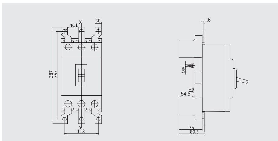
Z2Q: 插入式板前接线（三极）（X-X、Y-Y为断路器中心）
