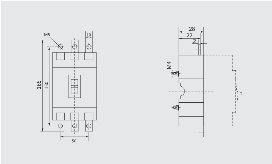
Z2Q：插入式板前接线（二极）（X-X、Y-Y为断路器中心）
