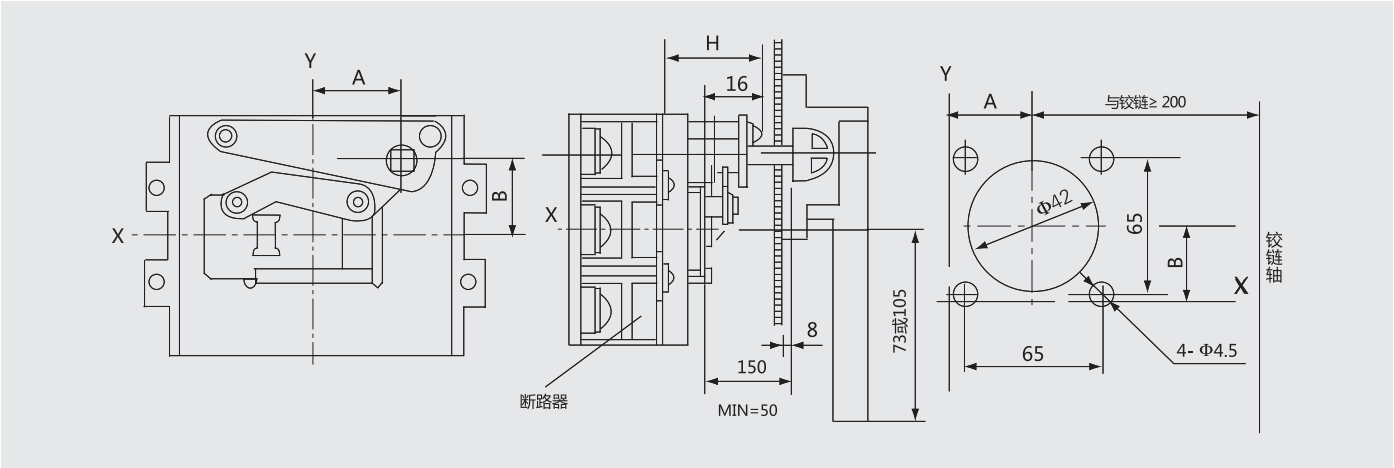
外形附件的安装方法及其外形尺寸
