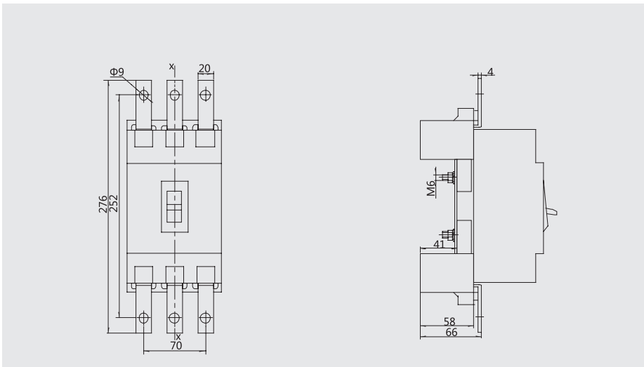
Z2Q：插入式板前接线（二极、三极）（X-X、Y-Y为断路器中心）
