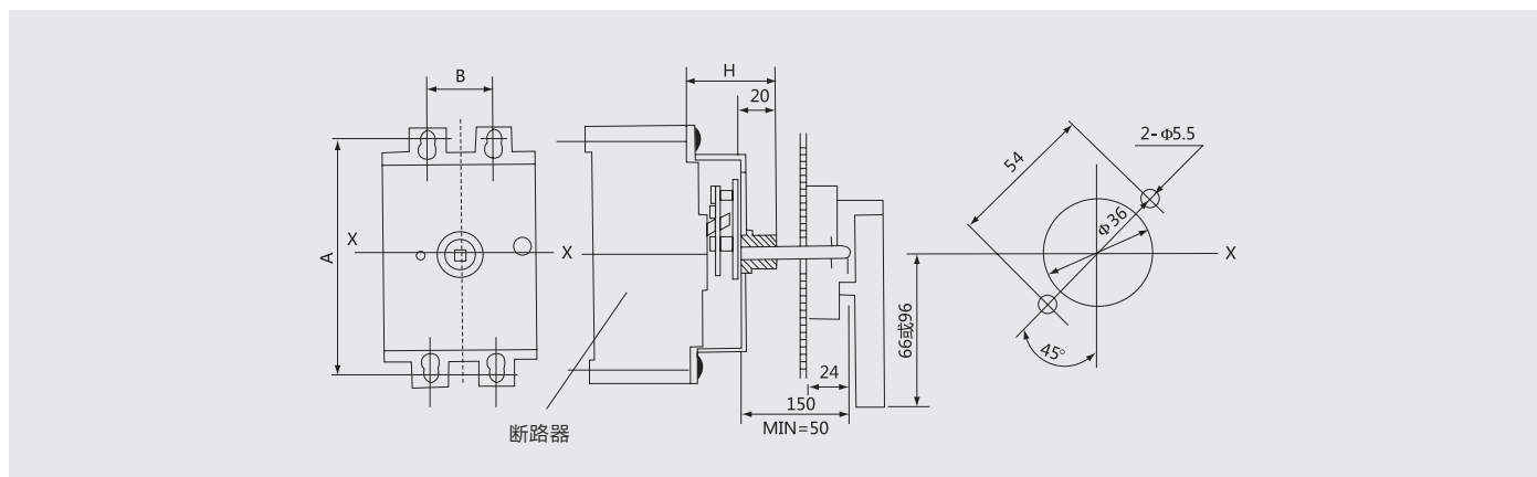
CS1-F型手柄安装开孔示意图
