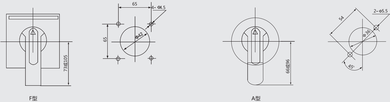
CSM2E 手动操作机构手柄安装开孔尺寸
