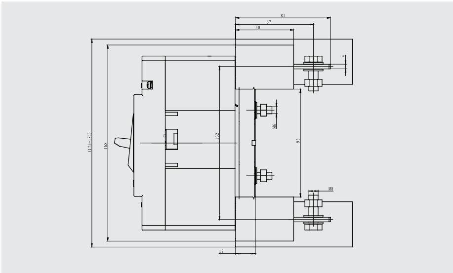
Z2H：插入式板后接线（二极、三极）（X-X、Y-Y为断路器中心）
