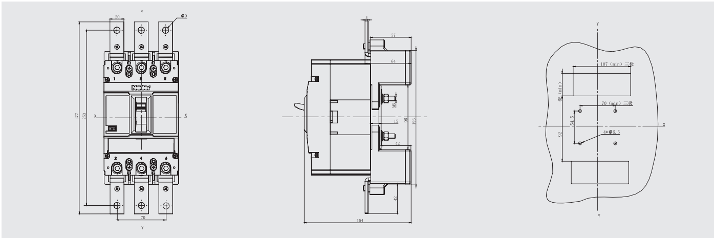
Z2Q：插入式板前接线（三极）
