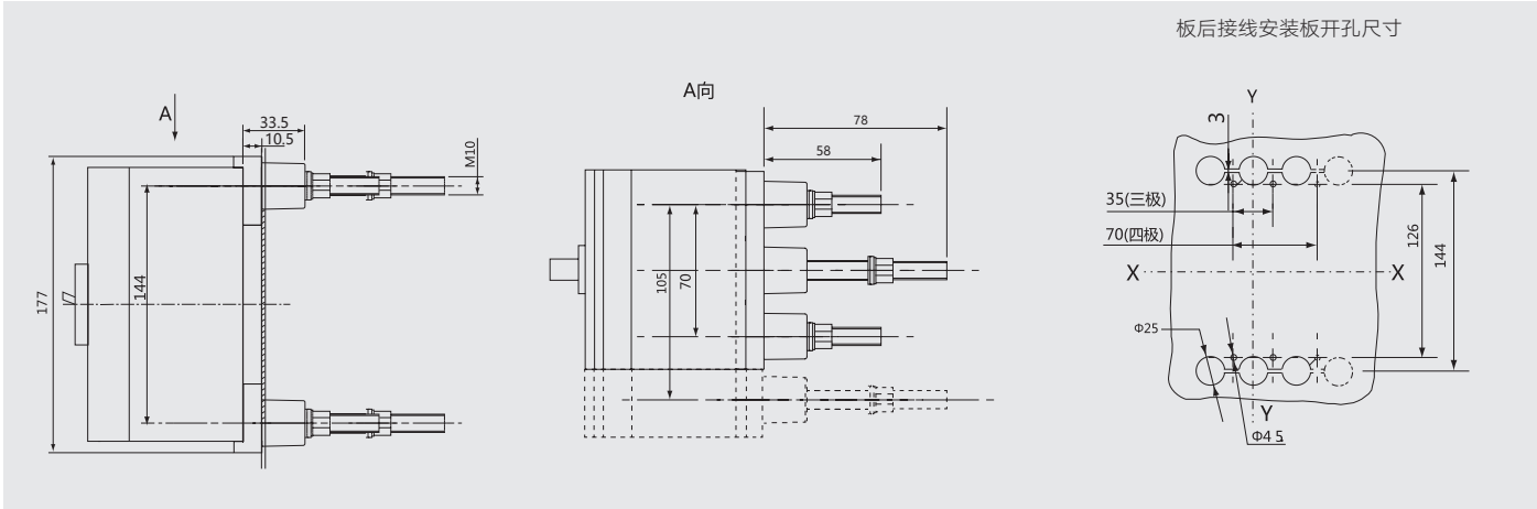
Z1：板后接线（三极、四极）（X-X、Y-Y为断路器中心）
