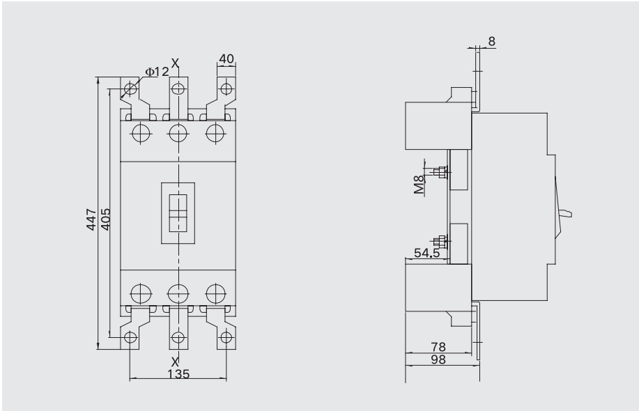
Z2Q：插入式板前接线（二极、三极）
