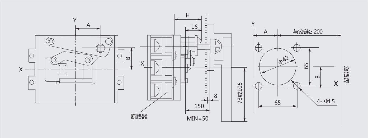
CS2-F型手柄安装开孔示意图
