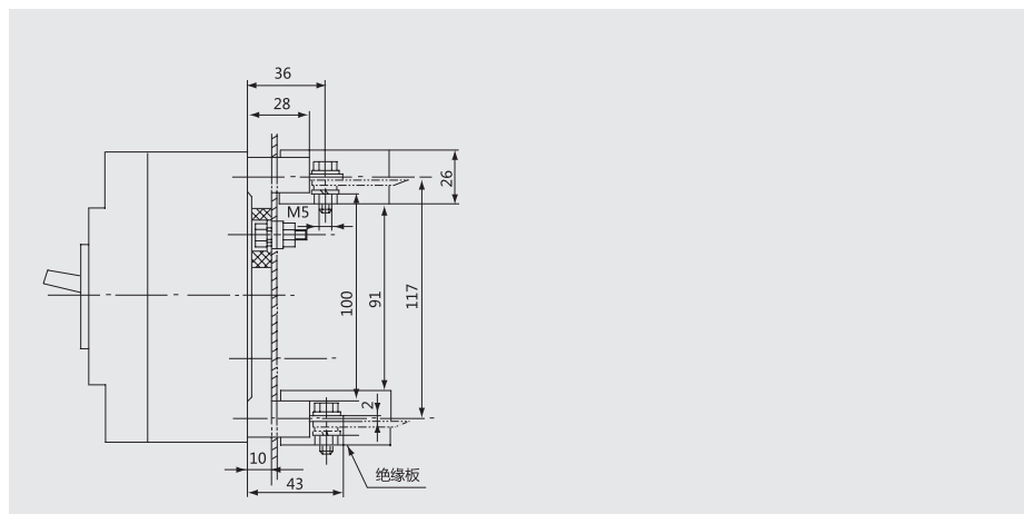
Z2H：插入式板后接线（三极、四极）（X-X、Y-Y为断路器中心）
