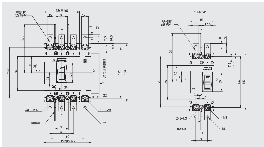
板前接线（二极、三极、四极）（X-X、Y-Y为三极断路器中心）
