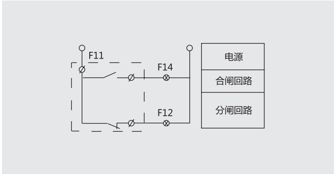
辅助触头接线图
