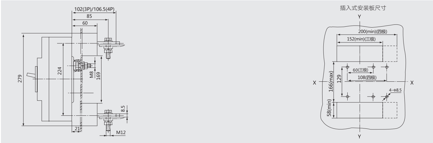
Z2H：插入式板后接线（三极、四极）（X-X、Y-Y为断路器中心）
