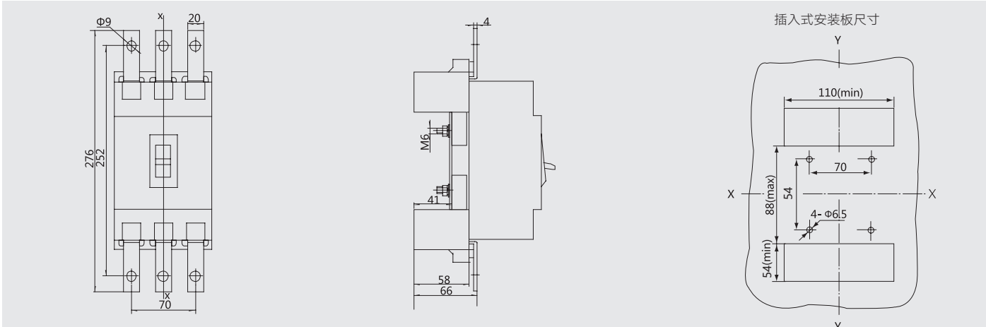
Z2Q：插入式板前接线（三极）（X-X、Y-Y为断路器中心）
