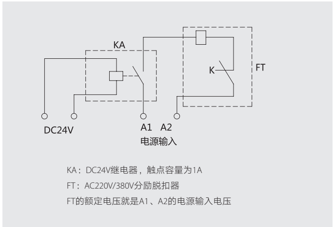
分励脱扣器瞬动电流及功耗
