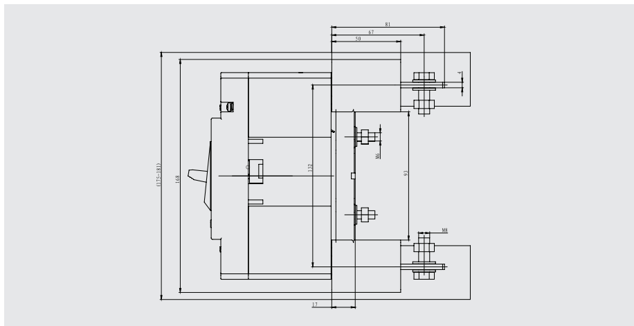
Z2H: 插入式板后接线 (二极、三极) (X-X、Y-Y为断路器中心)
