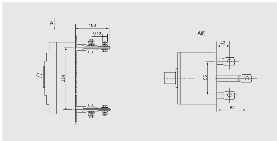
Z1: 板后接线（三极、四极）（X-X、Y-Y为断路器中心）
