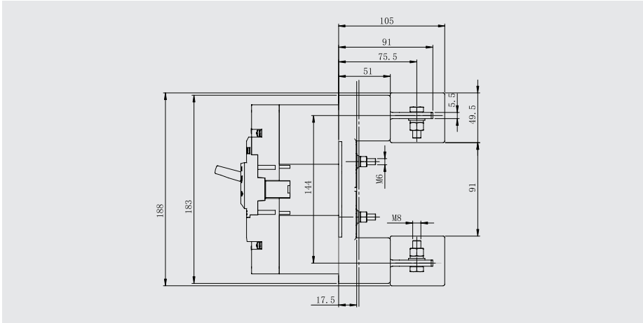
Z2H：插入式板后接线（三极）（X-X、Y-Y为断路器中心）
