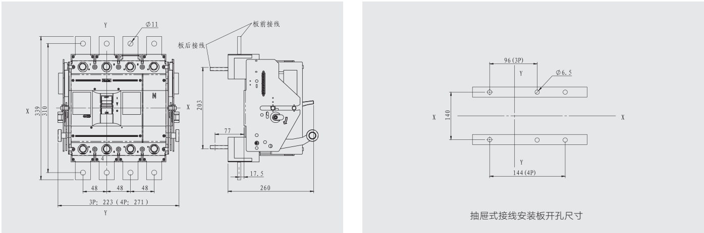
抽屉式接线（三极、四极）（X-X、Y-Y为三极断路器中心）
