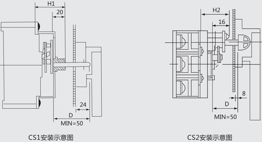
CSM2E 手动操作机构安装示意图
