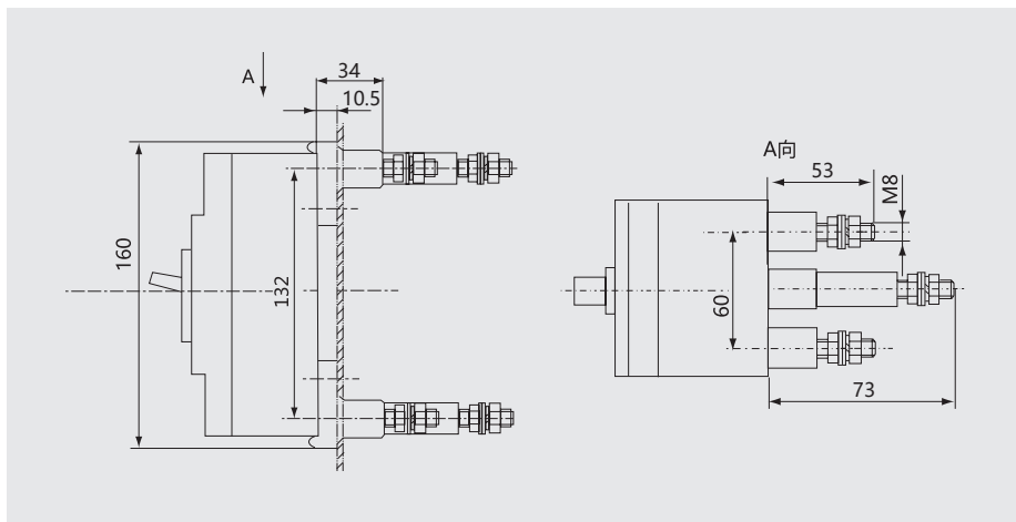
Z1: 板后接线 (二极、三极) (X-X、Y-Y 为断路器中心)
