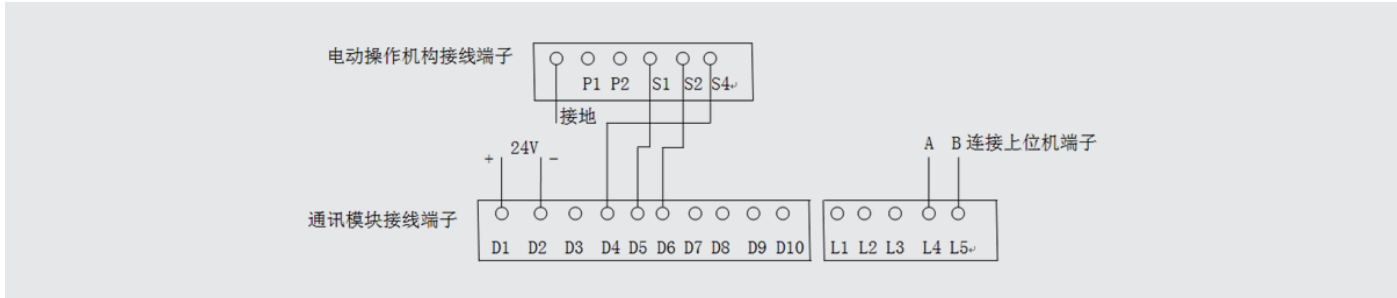
通讯模块与电操机构的连接图
